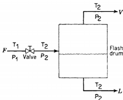
FIG. 13-16 Equilibrium flash separator.
